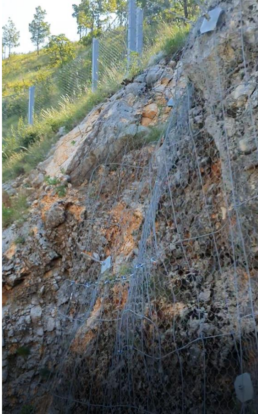
NEPROMIJENJENO STANJE; sanaciona mjera br. 8 (SN ankeri, čelična mreža velike čvrstoće i barijera po vrhu kosine)
