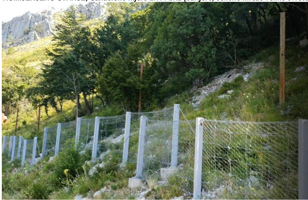
NEPROMIJENJENO STANJE; Sanaciona mjera br.3 (barijera od čelične mreže velike čvrstoće po vrhu kosine)
