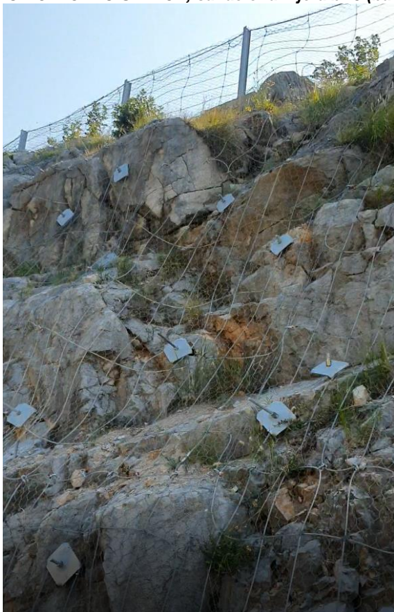
NEPROMIJENJENO STANJE; sanaciona mjera br.4 (barijera, SN ankeri, čelična mreža velike čvrstoće)
