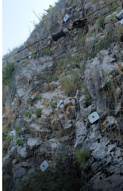
NEPROMIENJENO STANJE; Sanaciona mjera br.7 (barijera, SN ankeri, čelična mreža velike čvrstoće)
