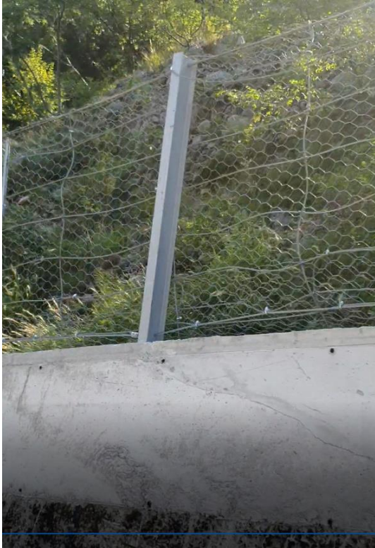
NEPROMIJENJENO STANJE; sanaciona mjera br.4 (nadvišenje zida i barijera od čelične mreže velike čvrstoće)
