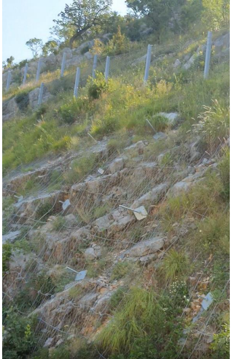
NEPROMIJENJENO STANJE; Sanacione mjere br.1 i br.2 (barijera, SN ankeri, čelična mreža velike čvrstoće)
