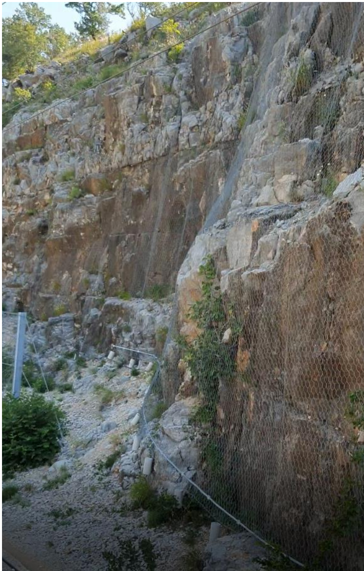
NEPROMIJENJENO STANJE; Sanaciona mjera br.6 (kosine prekrivene duplo uvijenom čeličnom mrežom i barijera od čelične mreže velike čvrstoće po vrhu kosine)
