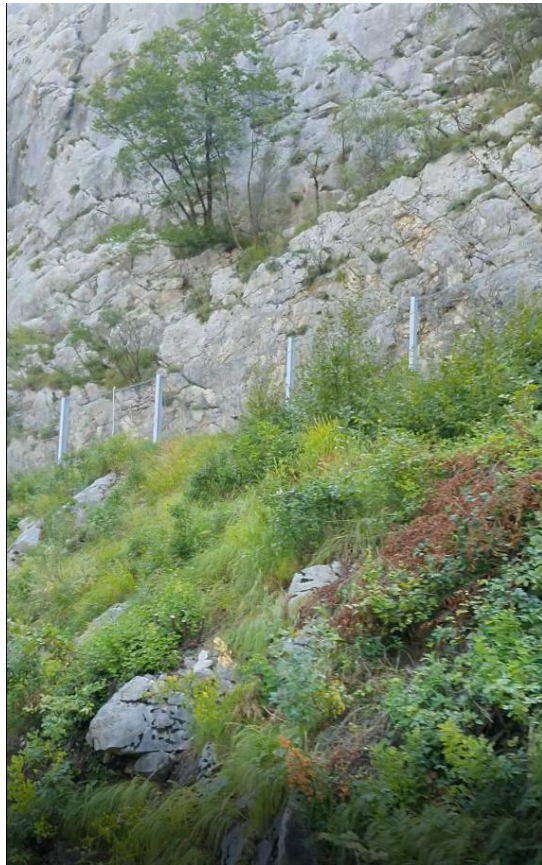
NEPROMIJENJENO STANJE; Sanaciona mjera br. 10 (u podnožju kosine postavljena barijera od čelične mreže velike čvrstoće)
