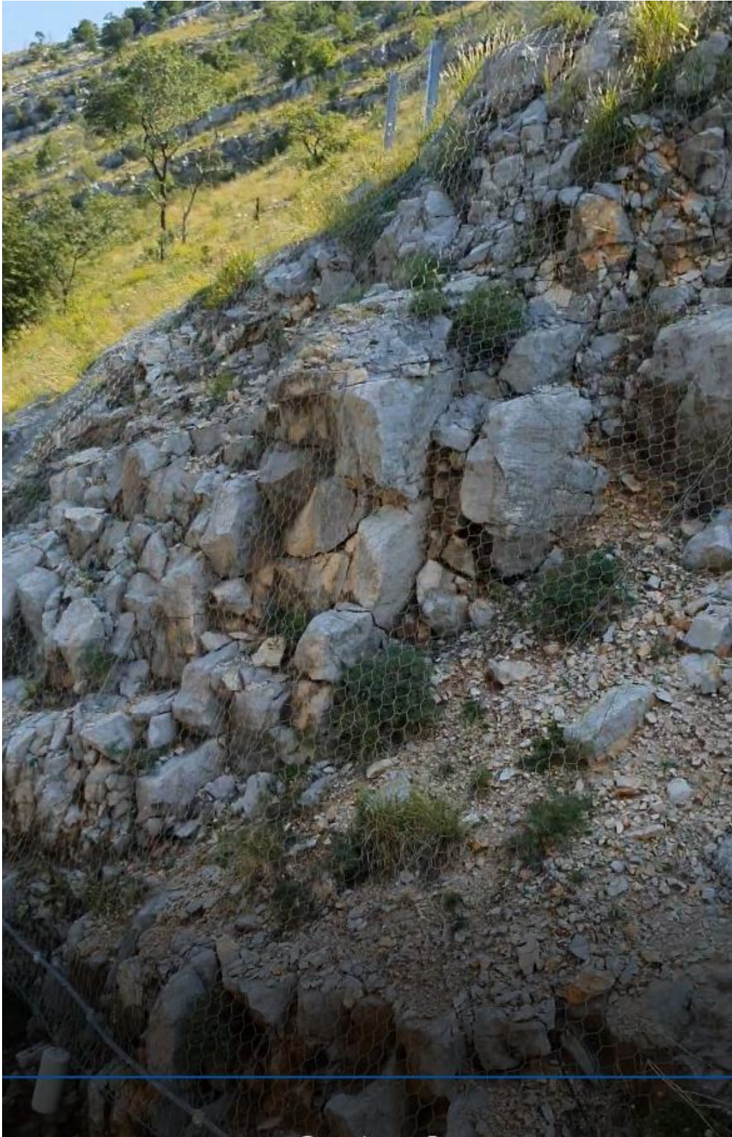
NEPROMIJENJENO STANJE; Sanaciona mjera br.4 (kosine prekrivene duplo uvijenom čeličnom mrežom i barijera od čelične mreže velike čvrstoće po vrhu kosine)
