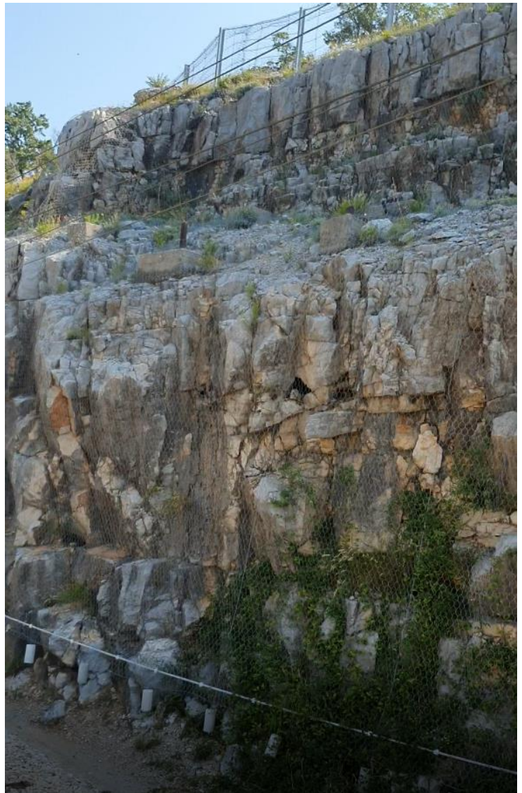
NEPROMIJENJENO STANJE; Sanaciona mjera br.6 (kosine prekrivene duplo uvijenom čeličnom mrežom i barijera od čelične mreže velike čvrstoće po vrhu kosine)
