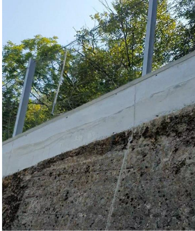
NEPROMIJENJENO STANJE; sanaciona mjera br.4 (nadvišenje zida i barijera od čelične mreže velike čvrstoće)
