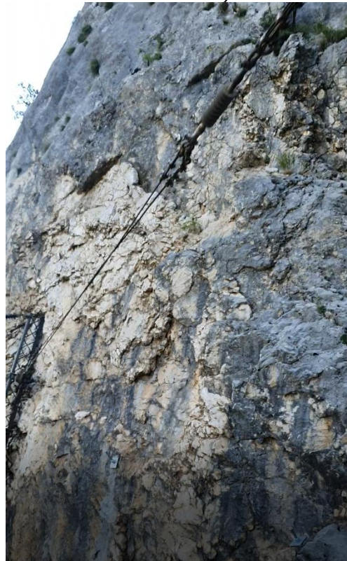
NEPROMIJENJENO STANJE; sanaciona mjera br. 9 (IBO ankeri ugrađeni na kritičnim mikrolokalitetima)
